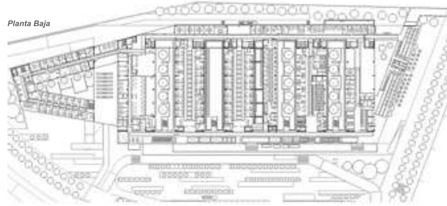
Planta Baja
